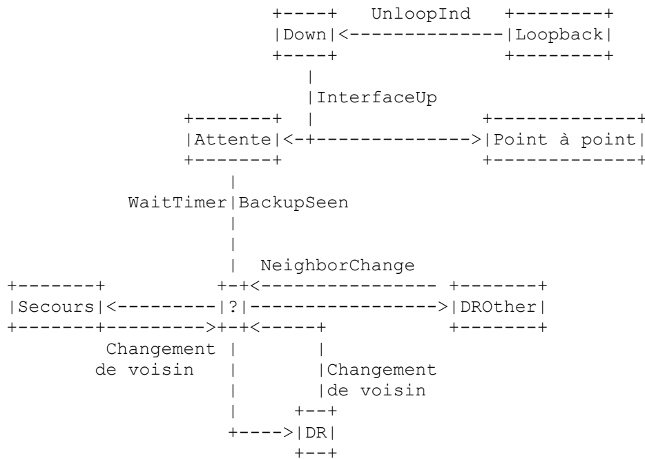
Figure 11 : Changements d'état d'interface
