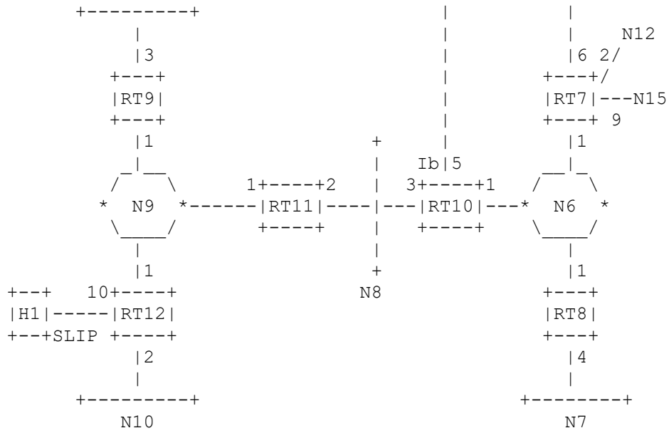
Figure 2 : Exemple de système autonome
