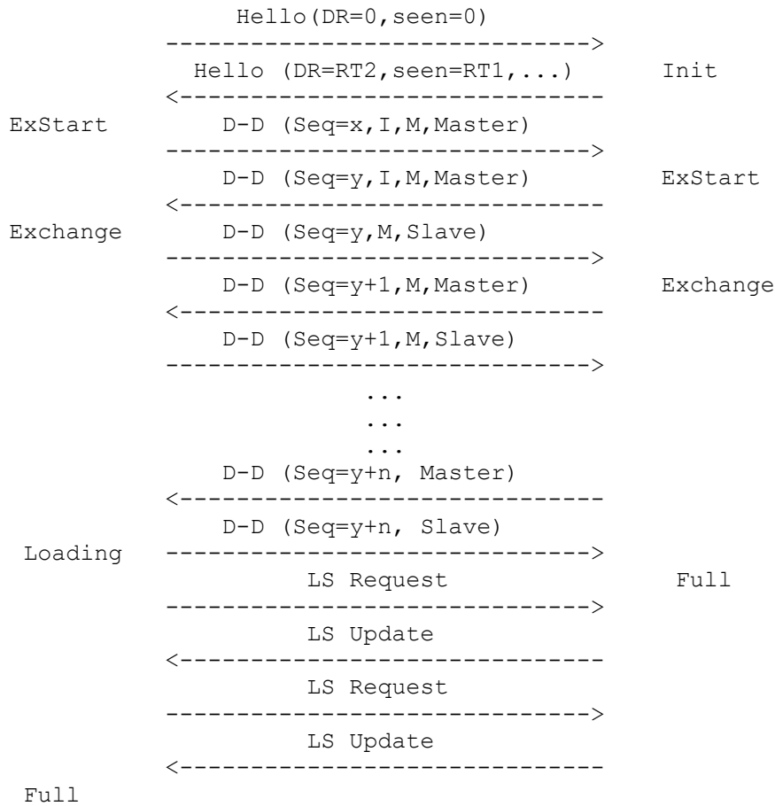
Figure 14 : Exemple de construction d'adjacence
