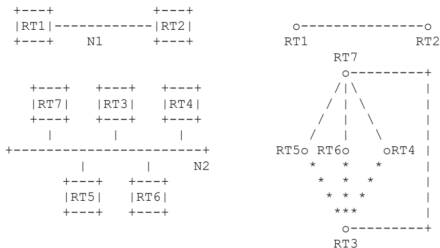
Figure 10 : Graphe des adjacences
