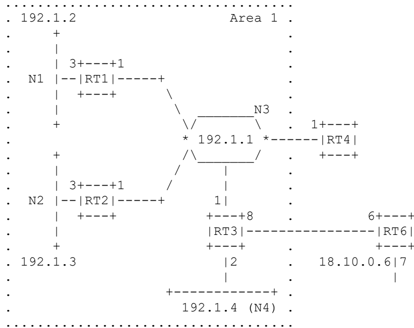
Figure 15 : Zone 1 avec indication des adresses IP
