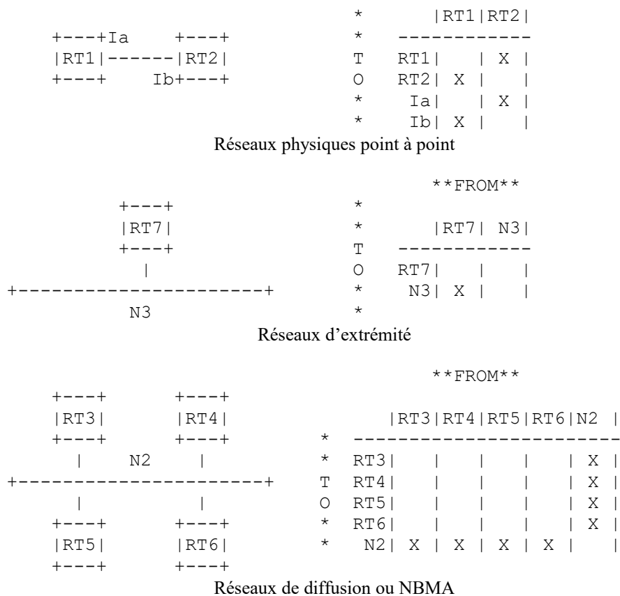
Figure 1a : Composants de cartographie de réseau
