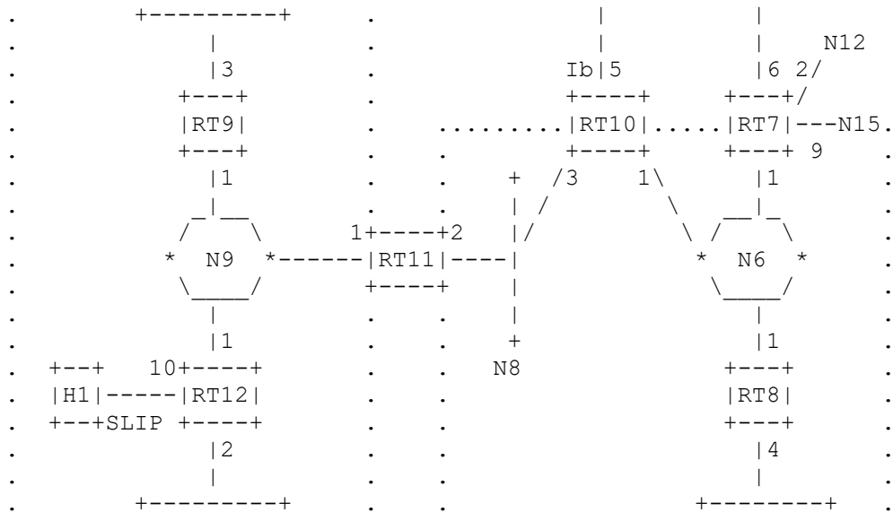
Figure 6 : Exemple de configuration de zone OSPF
