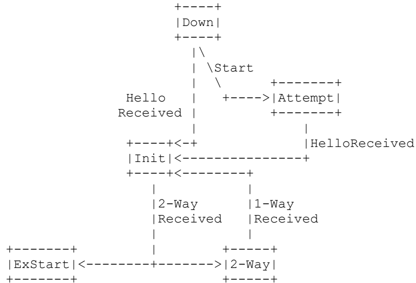
Figure 12 : Changements d'état du voisin (protocole Hello)
