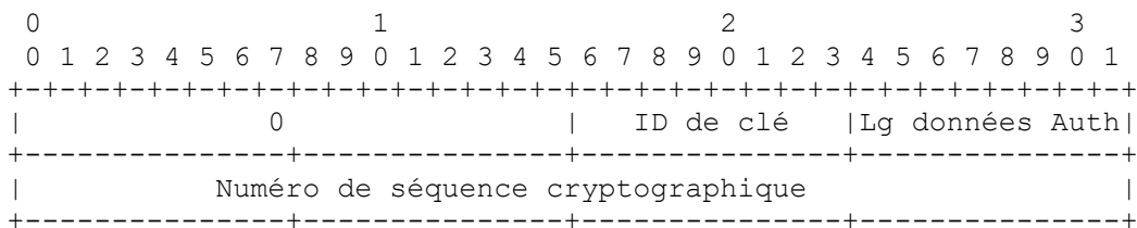
Figure 18 : Usage du champ Authentification dans l'en-tête de paquet OSPF lors de l'emploi de l'authentification cryptographique
