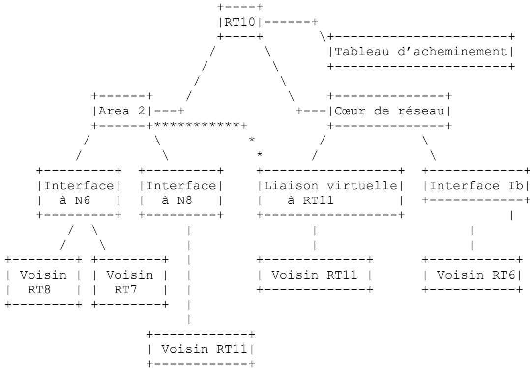
Figure 9 : Structure des données du routeur RT10
